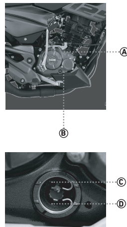
A: Tapón de aceite B: Visor medidor nivel de aceite C: Nivel superior D: Nivel inferior
